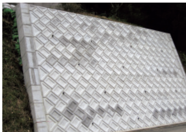
小口止ブロック+積ブロック（滑面タイプ）
