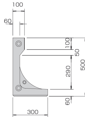
平面図
